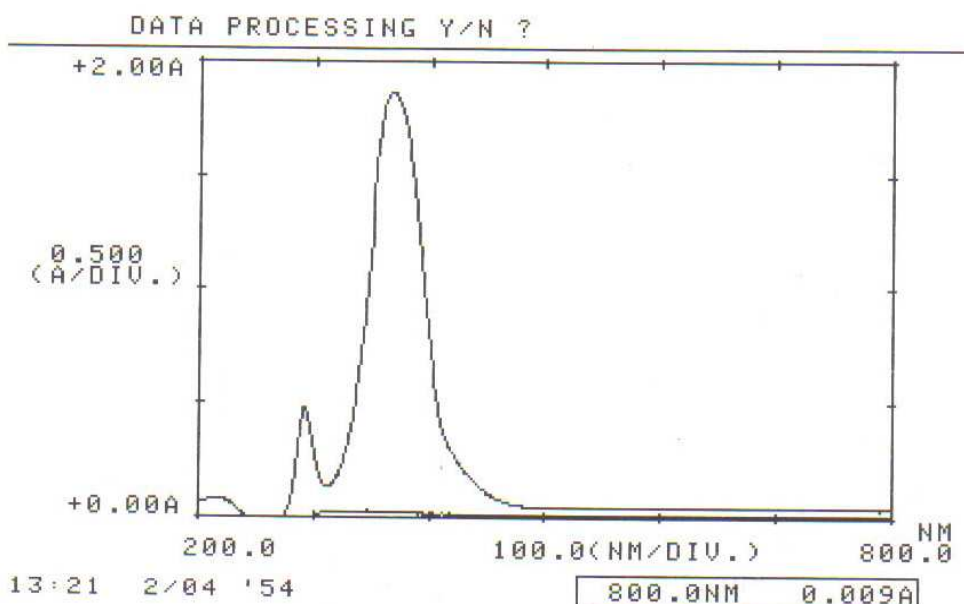
Figure 6 : Spectre UV de l'échantillon industriel (97 ppm en Cr(VI)) avant et après traitement avec le flocculant bio-organique
