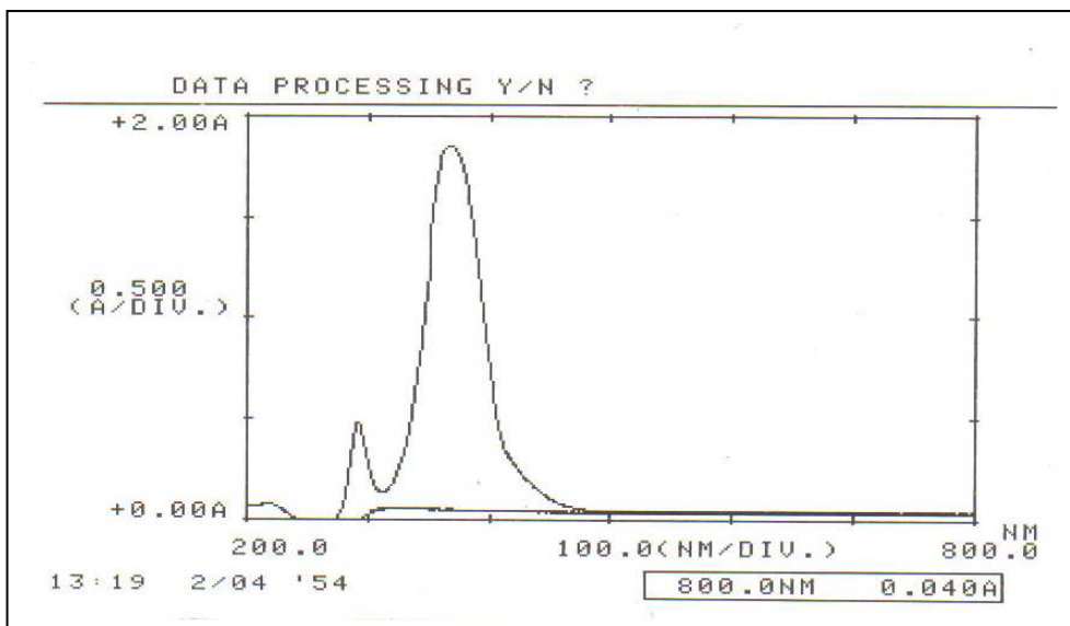
Figure 5 : Spectre UV de l'échantillon industriel (97 ppm en Cr(VI)) avant et après traitement avec le flocculant industriel
