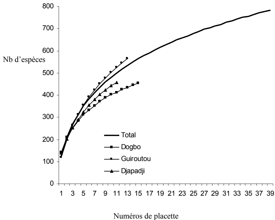
Figure 2 : Courbes aire-espèces des plantes inventoriées dans chaque secteur d'étude et dans l'ensemble du Sud-PNT.
